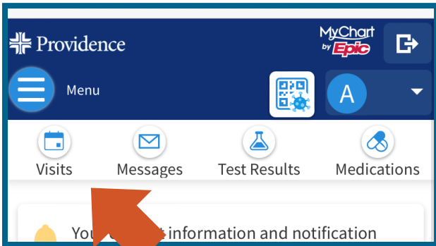
Browser
